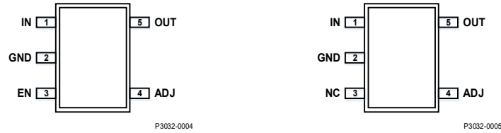
图4.3 SOT23-5封装 注2 (2.92mm×2.8mm×1.1mm)
