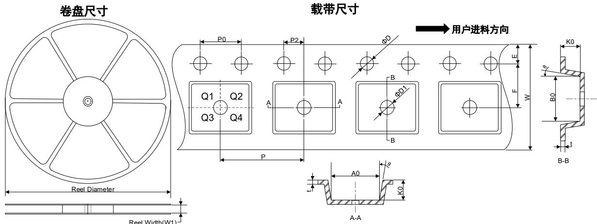
卷盘尺寸
